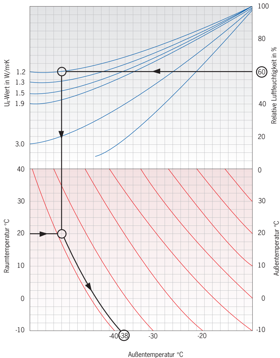
Taupunkt Diagramm (nach DIN 4701)
